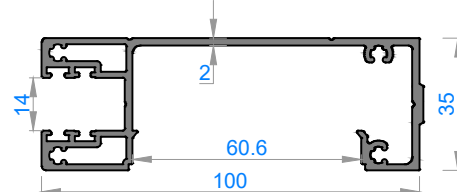
Sistem Kodu 6116* Ağırlık (kg/mt) 1,541
