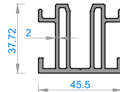
5028 TAKOZ KESİM ÖLÇÜLERİ
