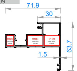
Sistem Kodu 6121* Ağırlık (kg/mt) 0,067
