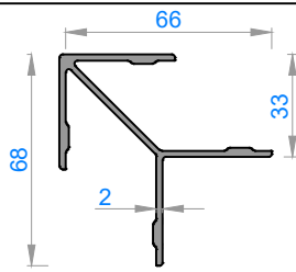
270 TAKOZ KESİM ÖLÇÜLERİ
