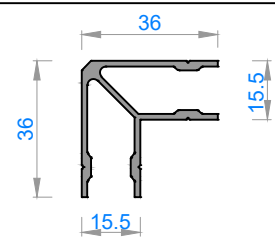
275 TAKOZ KESİM ÖLÇÜLERİ
