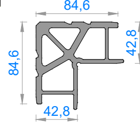
4951 TAKOZ KESİM ÖLÇÜLERİ
