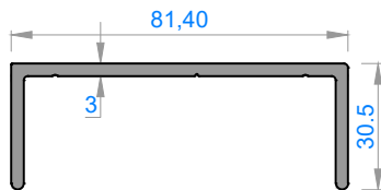
5509 TAKOZ KESİM ÖLÇÜLERİ
