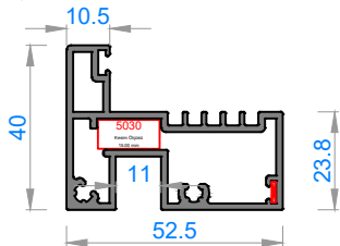
Sistem Kodu 6115* Ağırlık (kg/mt) 0,201
