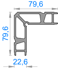
4950 TAKOZ KESİM ÖLÇÜLERİ
