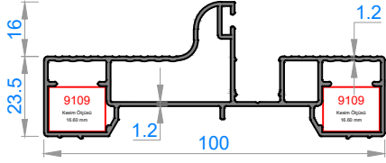
Sistem Kodu 6103 Ağırlık (kg/mt) 0,281
